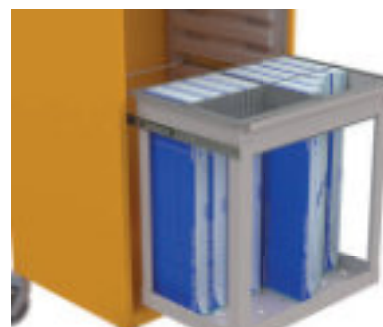
Support télescopique pour sondes emballées
